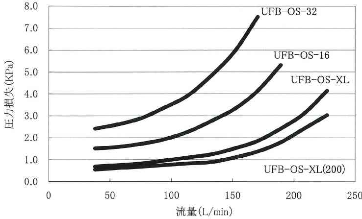
UFB-OS-シリーズ 圧力損失グラフ
